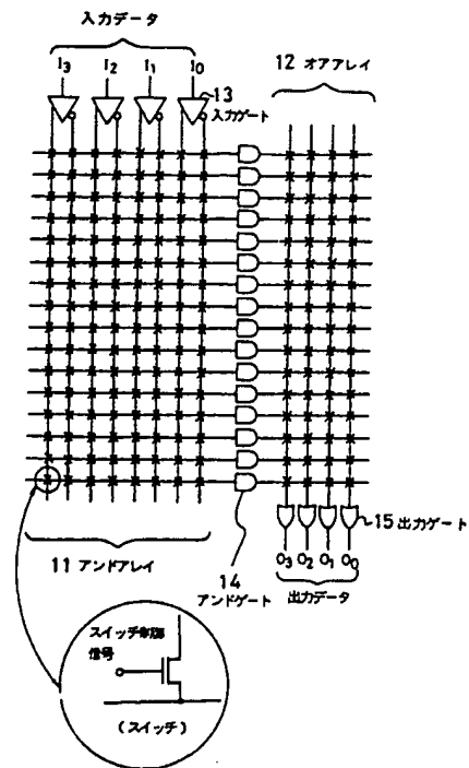
プログラマブル論理アレイ10の回路図 第3図
